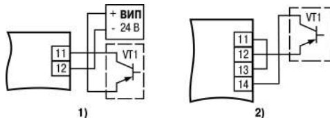
Рисунок 5.4 – Подключение дискретных датчиков с п-п-выходом: 1) при работе датчика от ВИП; 2) при работе датчика от внутреннего источника питания
