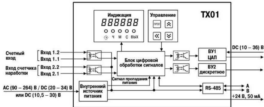
Рисунок 6.1 – Функциональная схема прибора
